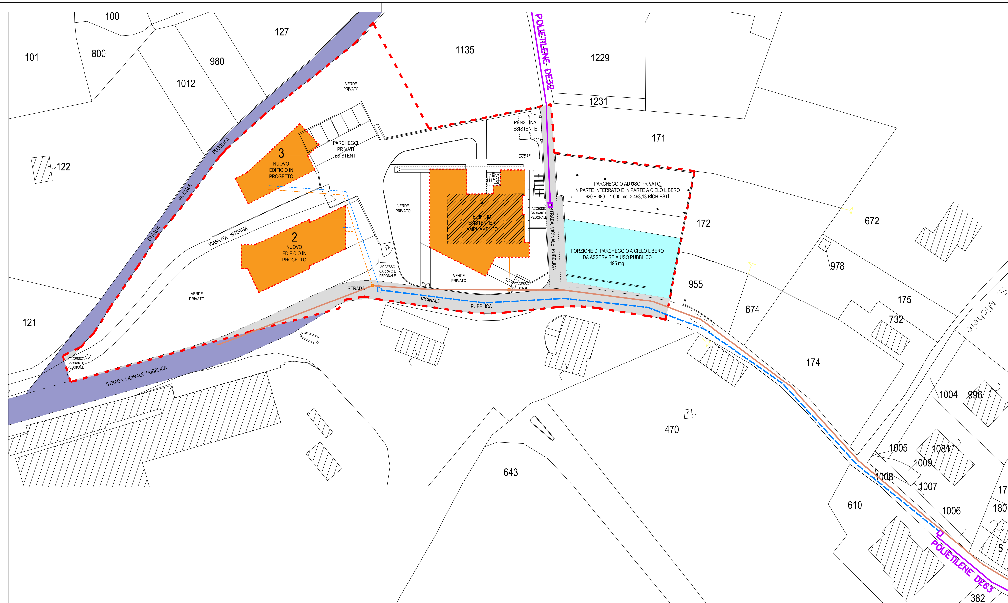
PLANIMETRIA P.E.C IN VARIANTE CON INDIVIDUAZIONE DELLE OPERE DI URBANIZZAZIONE
