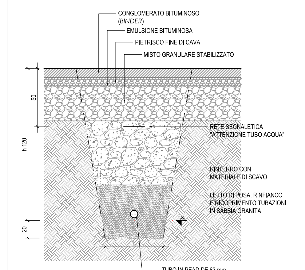
PARTICOLARI COSTRUTTIVI RETE ACQUEDOTTO
