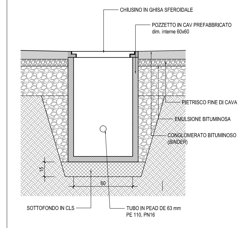
PARTICOLARI COSTRUTTIVI RETE ACQUEDOTTO
